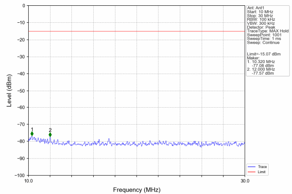
10MHz-30MHz
