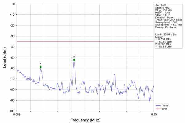
9kHz-150kHz
