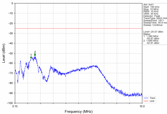
150kHz-10MHz
