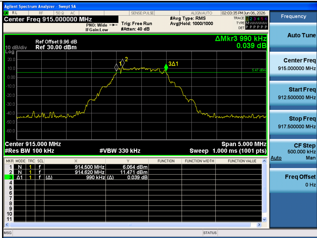
LORA_OFDM_LR-Ant1-915-PASS
