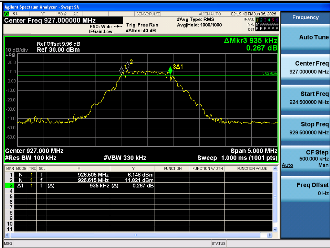
LORA_OFDM_LR-Ant1-927-PASS
