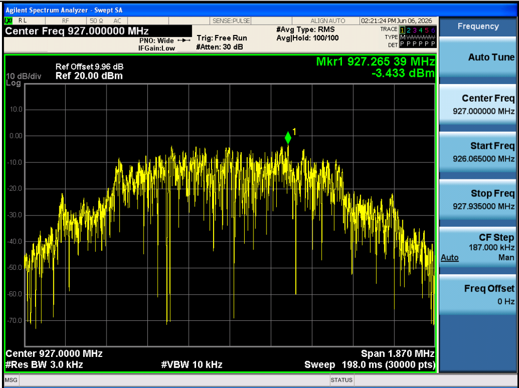
LORA_OFDM_LR-Ant1-927-PASS
