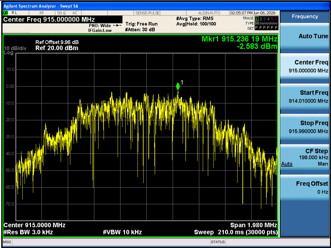
LORA_OFDM_LR-Ant1-915-PASS
