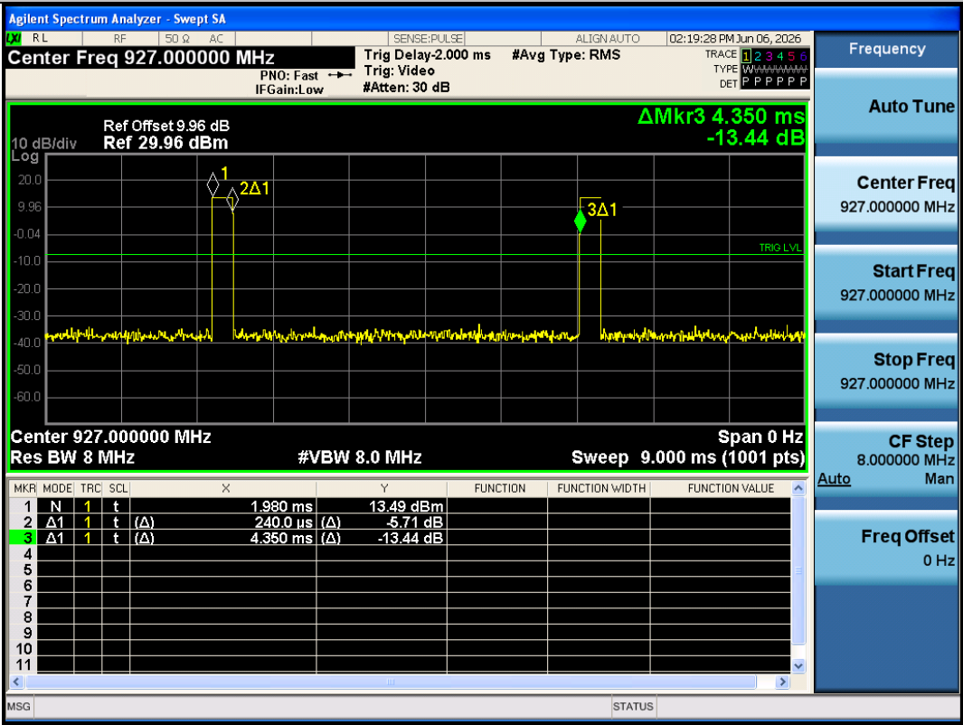
NTNV-LORA_OFDM_LR-Ant1-927
