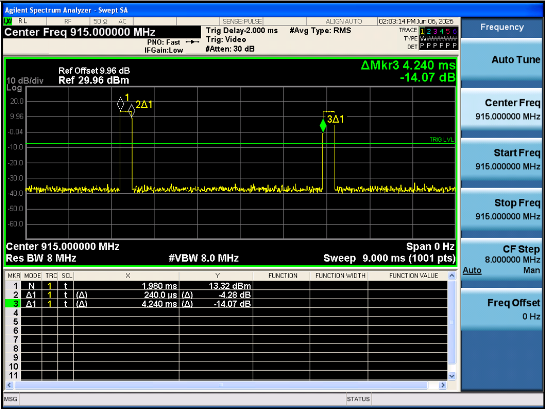
NTNV-LORA_OFDM_LR-Ant1-915
