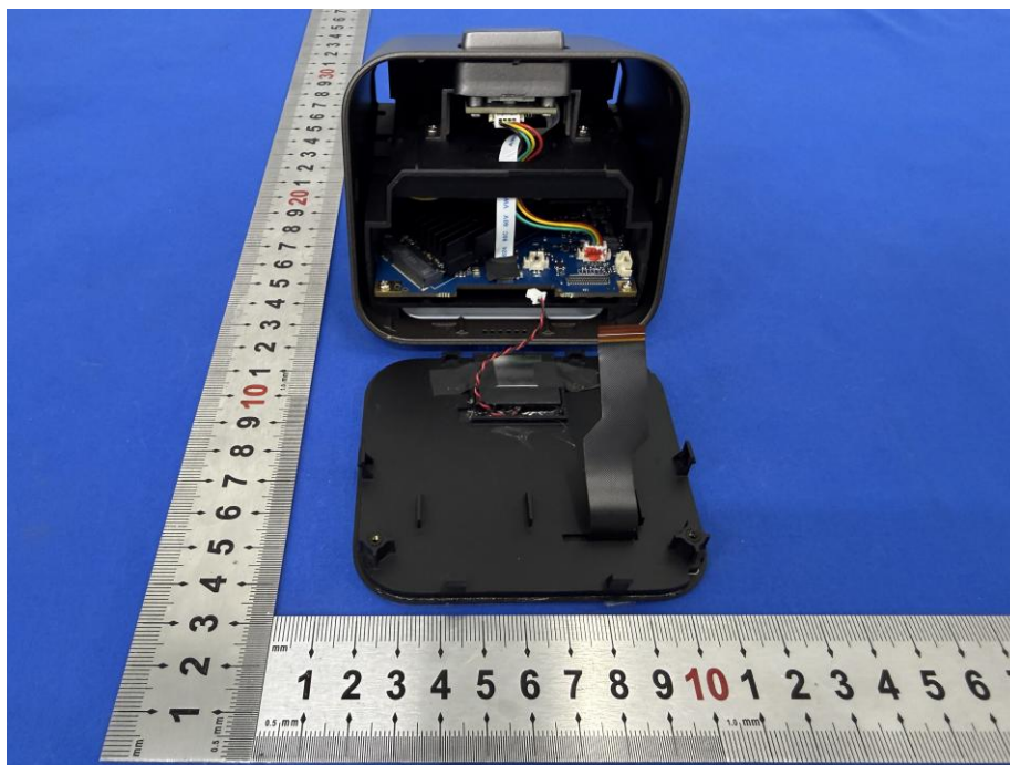
BT/WIFI Antenna
