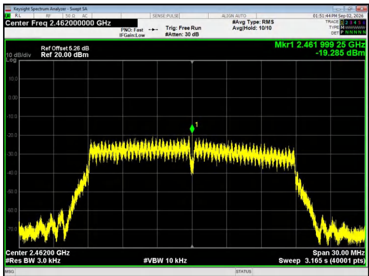
802.11ax20 - CH11
