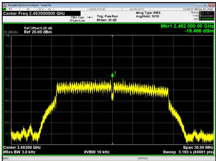
802.11g - CH11
