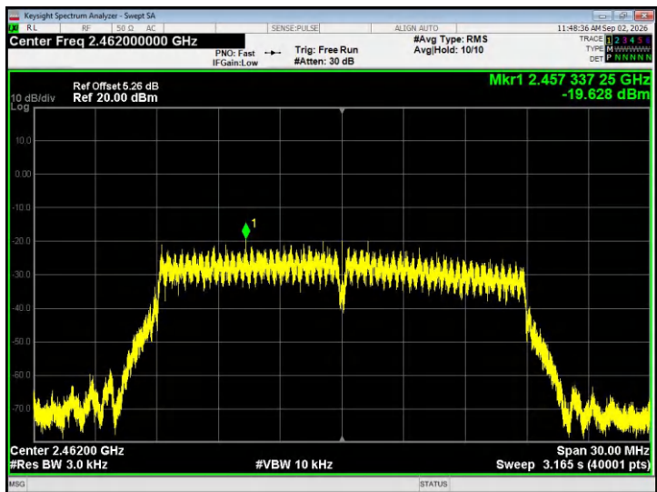
802.11n20 - CH11
