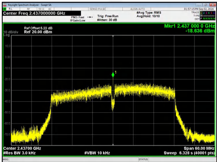
802.11ax40 - CH06
