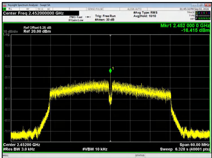
802.11n40 - CH09
