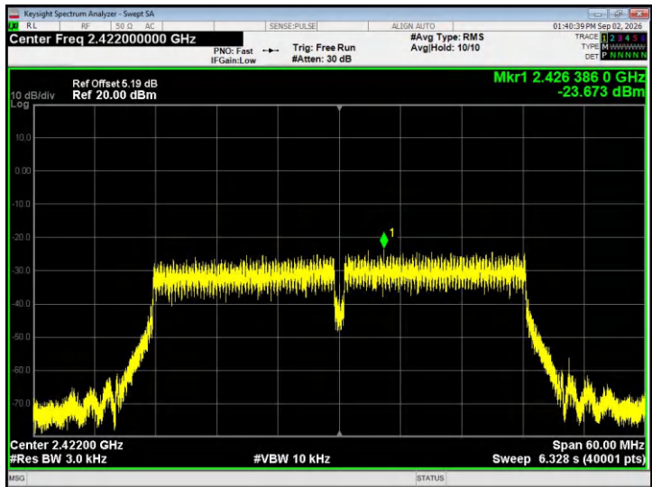
802.11n40 - CH03
