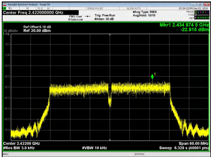
802.11ax40 - CH03
