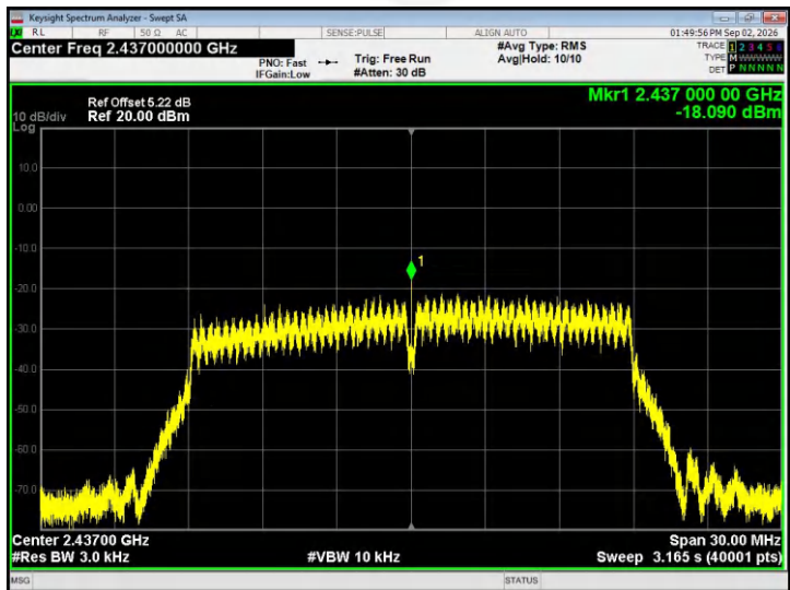
802.11ax20 - CH06
