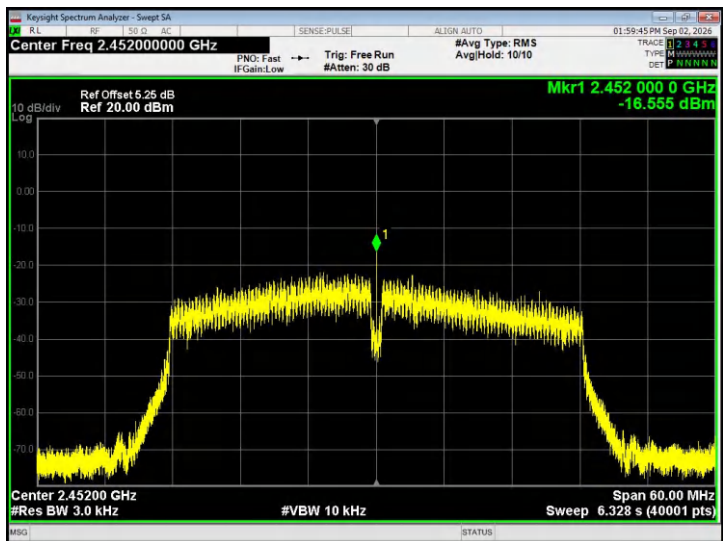
802.11ax40 - CH09
