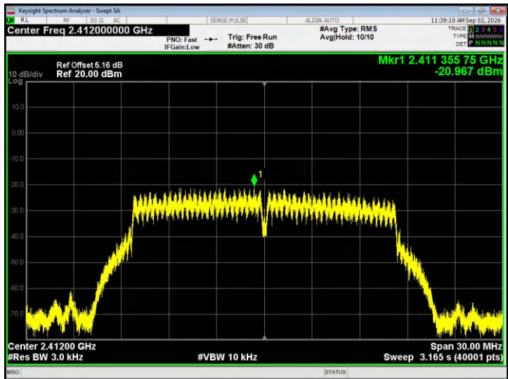
802.11g - CH01
