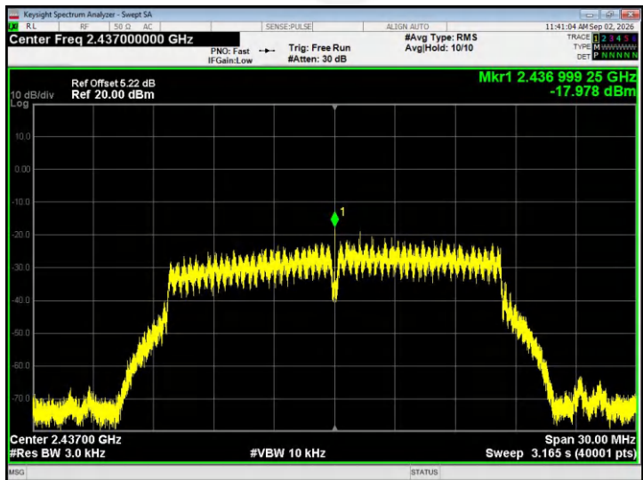
802.11g - CH06
