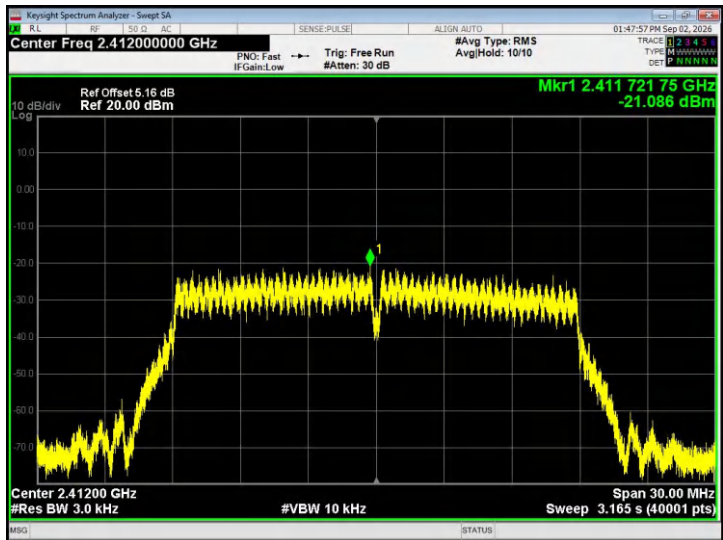
802.11ax20 - CH01
