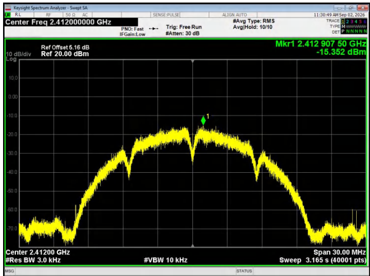
802.11b - CH01
