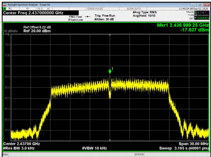
802.11n20 - CH06
