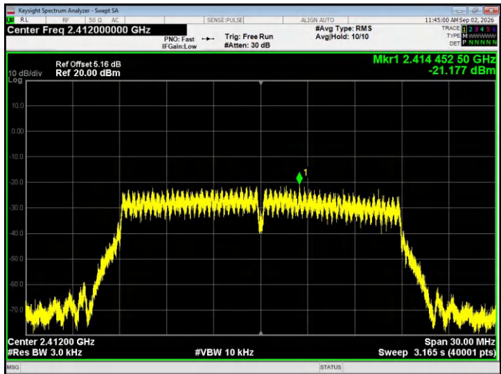
802.11n20 - CH01
