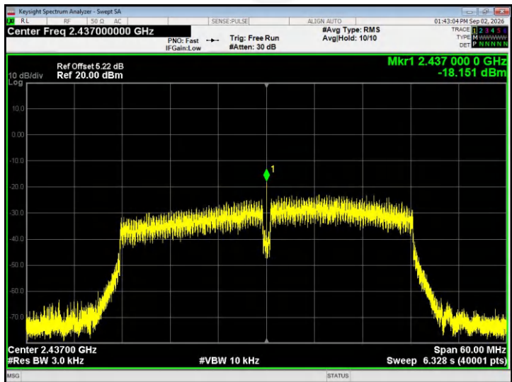
802.11n40 - CH06
