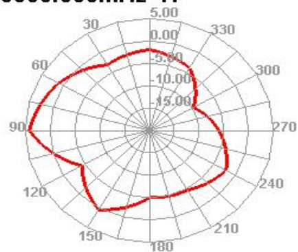
5500.000MHz H
