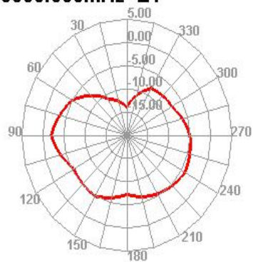
5500.000MHz E1
