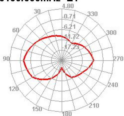
5150.000MHz E1
