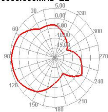
5500.000MHz E2
