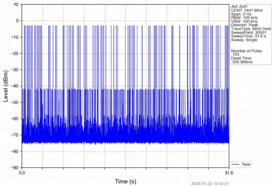
GFSK_DH5_HOPP_ANT_NTNV
