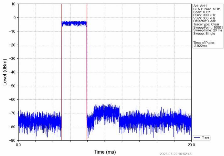
GFSK_DH5_HOPP_ANT_NTNV
