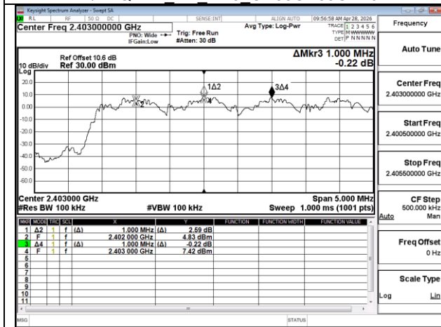
8DPSK 3M DH5 CH0CH1CH2
