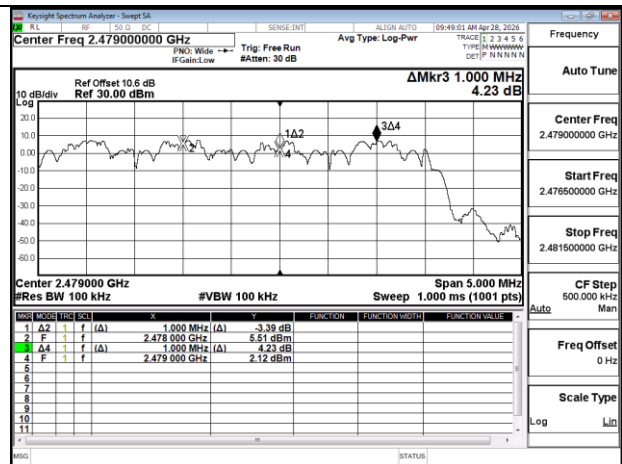
\pi/4 DQPSK 2M DH5 CH76CH77CH78
