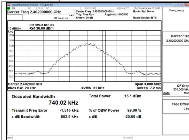
OBW 20dB GFSK 1M DH5 2402MHz
