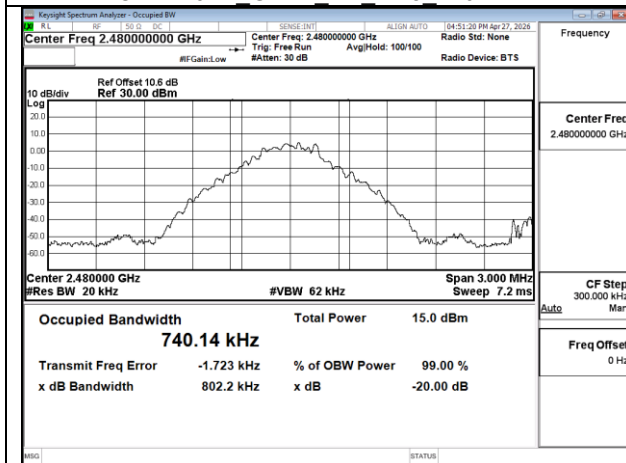
OBW 20dB GFSK 1M DH5 2480MHz
