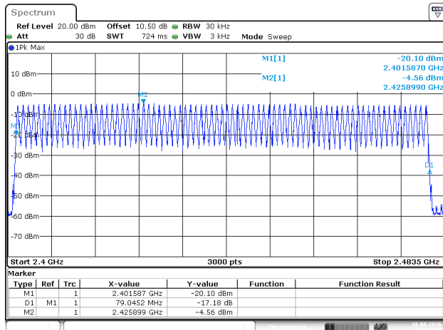
DH1_Hopping
