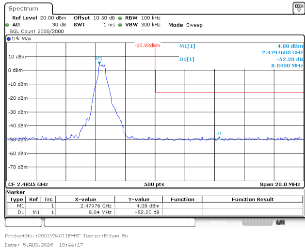
DH1_Hopping_Upper
