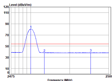
BLE_1M_TX_CH_39_Horizontal-AVG
