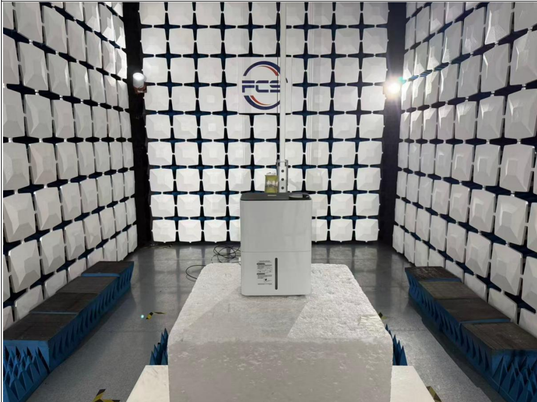
RE(Above 1GHz)
