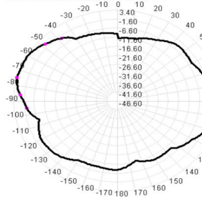
2400.0MHz Total(E1-XZ), Max= 3.40dBi
