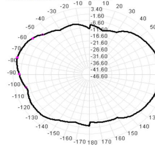
2400.0MHz Total(E2-YZ), Max= 2.21dBi
