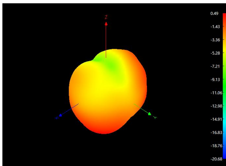
2500MHz 3D
