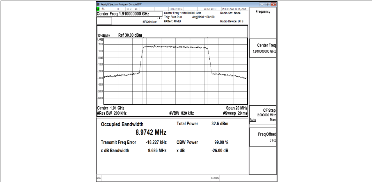
Band25-10MHz-QPSK-26640-50RB#0-PASS
