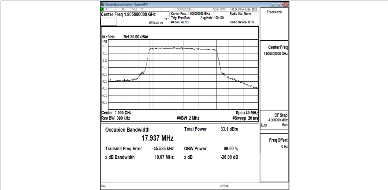
Band25-20MHz-QPSK-26590-100RB#0-PASS
