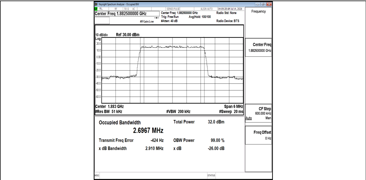
Band25-3MHz-QPSK-26365-15RB#0-PASS
