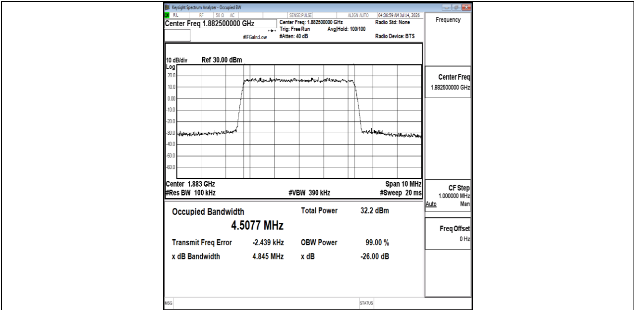
Band25-5MHz-QPSK-26365-25RB#0-PASS
