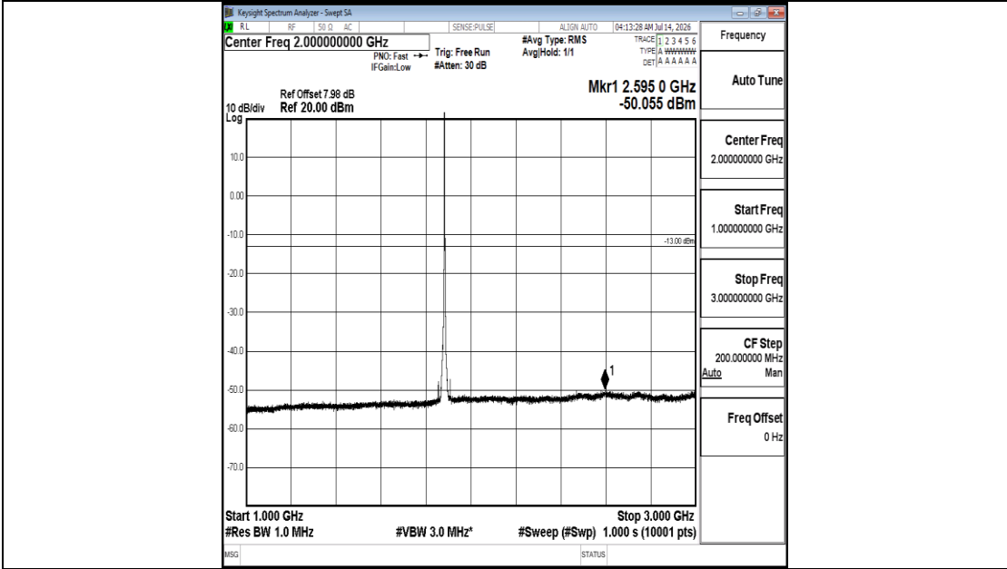
Band25-3MHz-QPSK-26365-1RB#0-1000~3000-PASS
