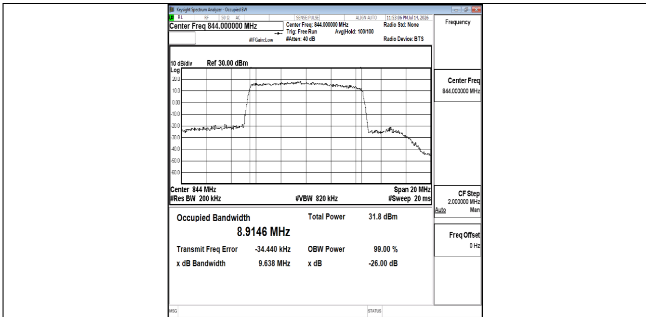
Band26(824-849)-10MHz-QPSK-26990-50RB#0-PASS
