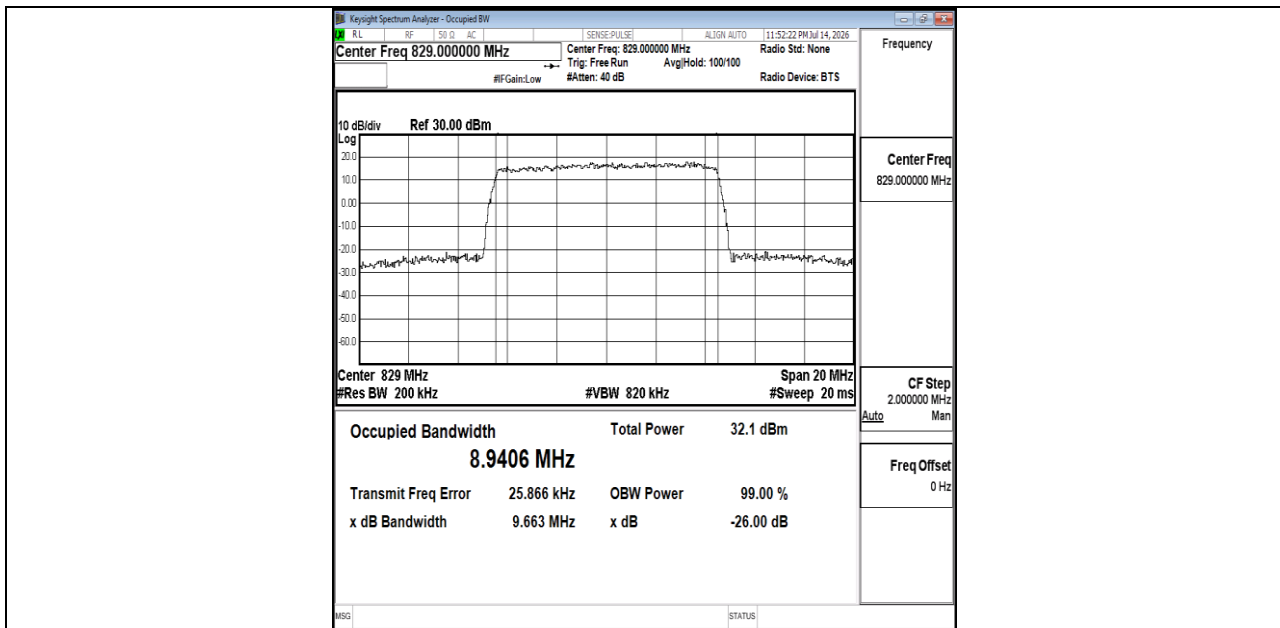
Band26(824-849)-10MHz-QPSK-26840-50RB#0-PASS
