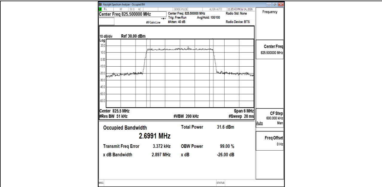
Band26(824-849)-3MHz-QPSK-26805-15RB#0-PASS
