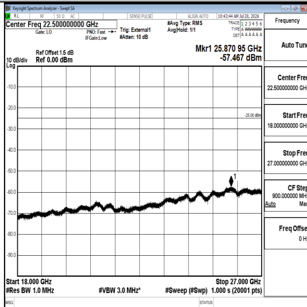
Band41-20MHz-16QAM-41490-1RB#0-18000~27000-PASS
