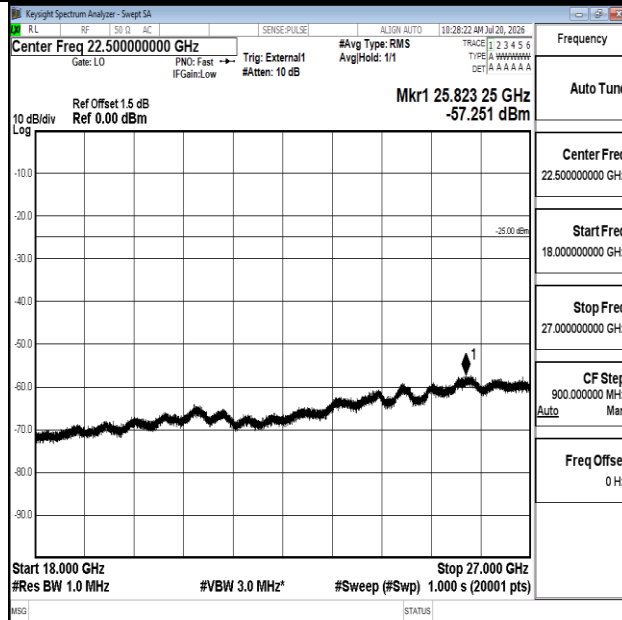
Band41-15MHz-16QAM-41515-1RB#0-18000~27000-PASS
