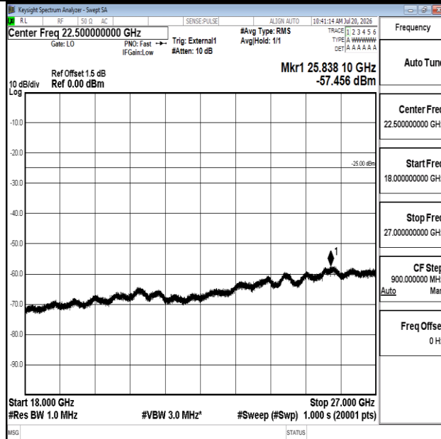
Band41-20MHz-QPSK-41490-1RB#0-18000~27000-PASS
