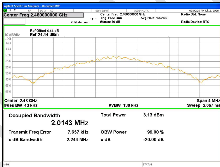
-20dB Bandwidth 2480MHz Ant1
