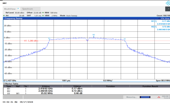
11N40SISO_Ant1_2437
