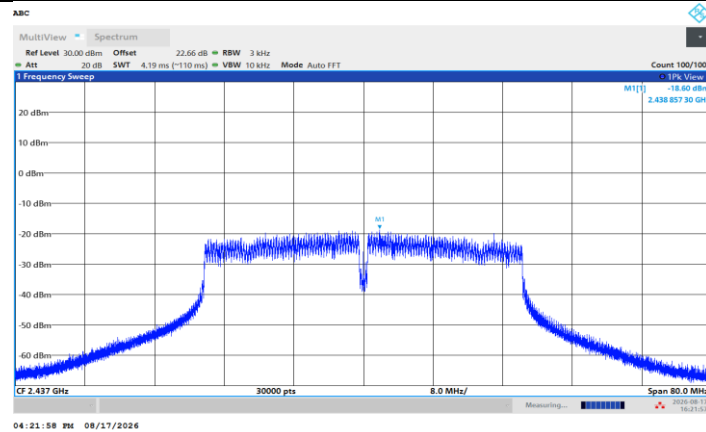
11N40SISO_Ant1_2437
