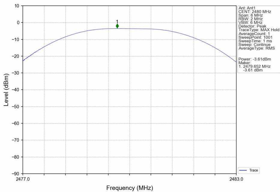
Peak Power NVNT BLE 2M 2480MHz Ant1
