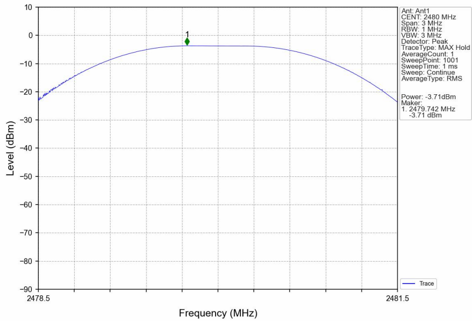
Peak Power NVNT BLE 1M 2480MHz Ant1
