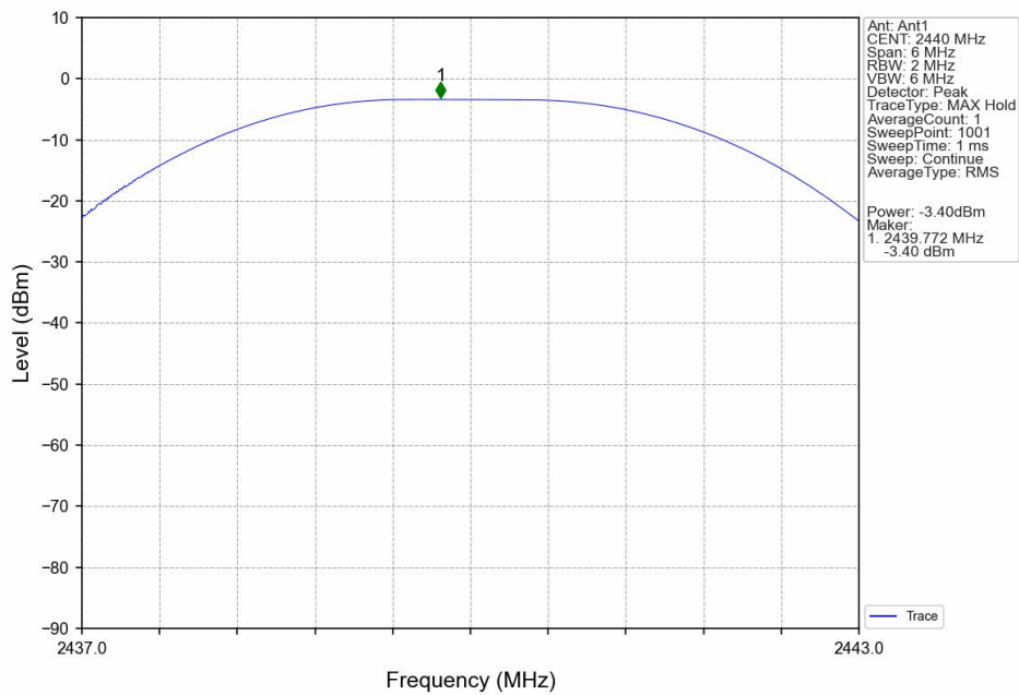
Peak Power NVNT BLE 2M 2440MHz Ant1
