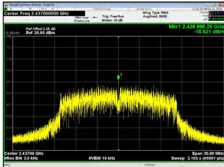
802.11g - CH06
