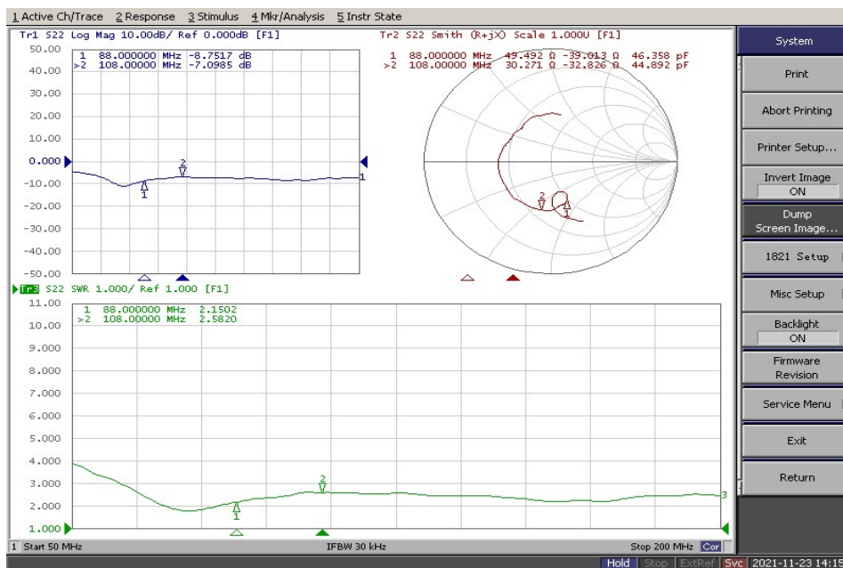
VSWR:
