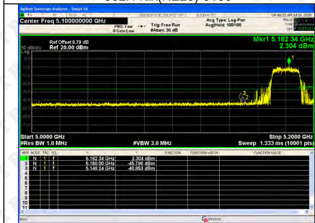
802.11ax(HE20)-5180
