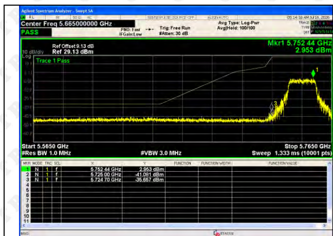
802.11(n40)-5755
