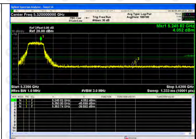
802.11n(HT40)-5230
