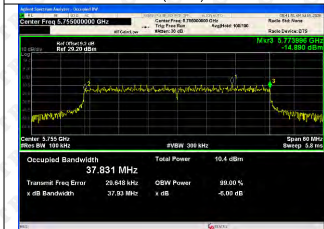
802.11ax(HE40)-5755
