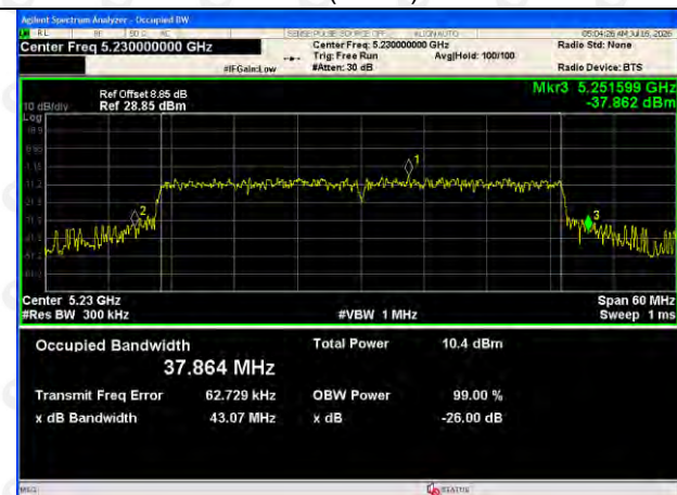
802.11ax(HE40)-5230
