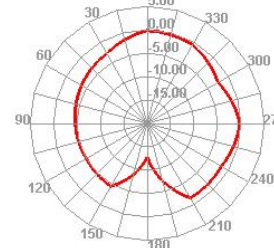
2690.000MHz E1
