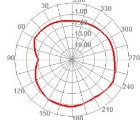
2690.000MHz E2
