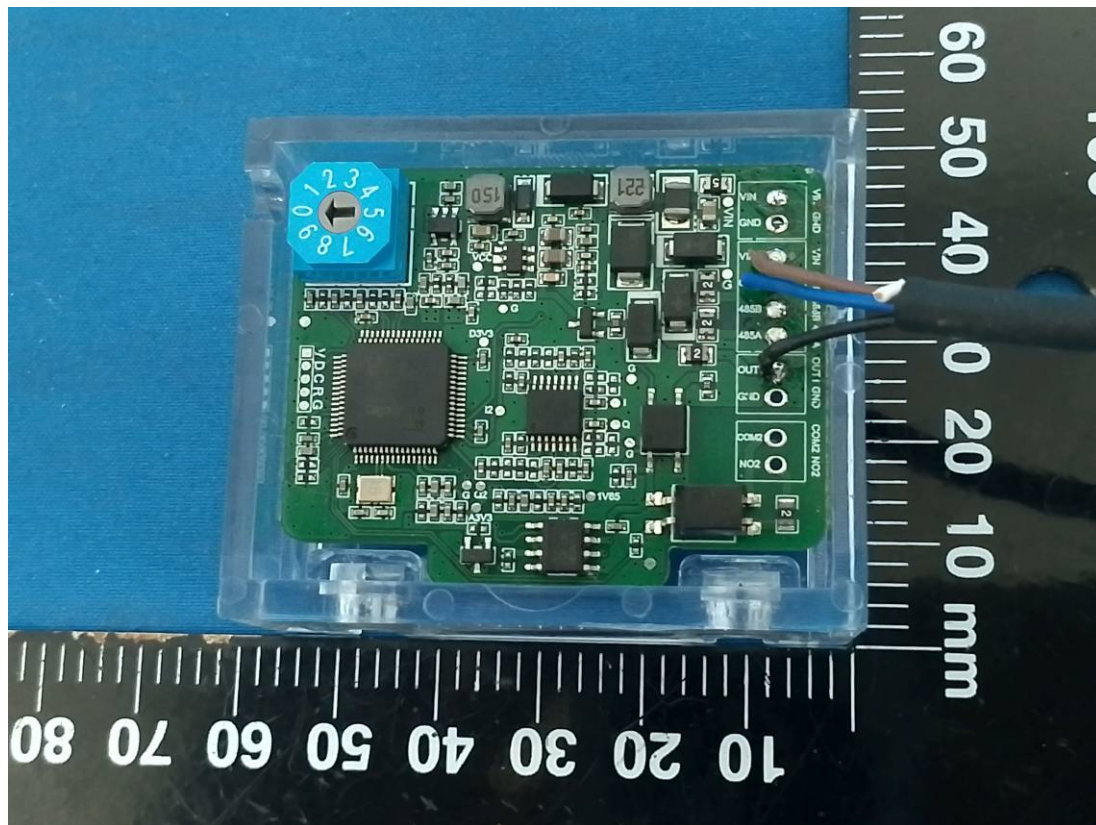
coding switch
