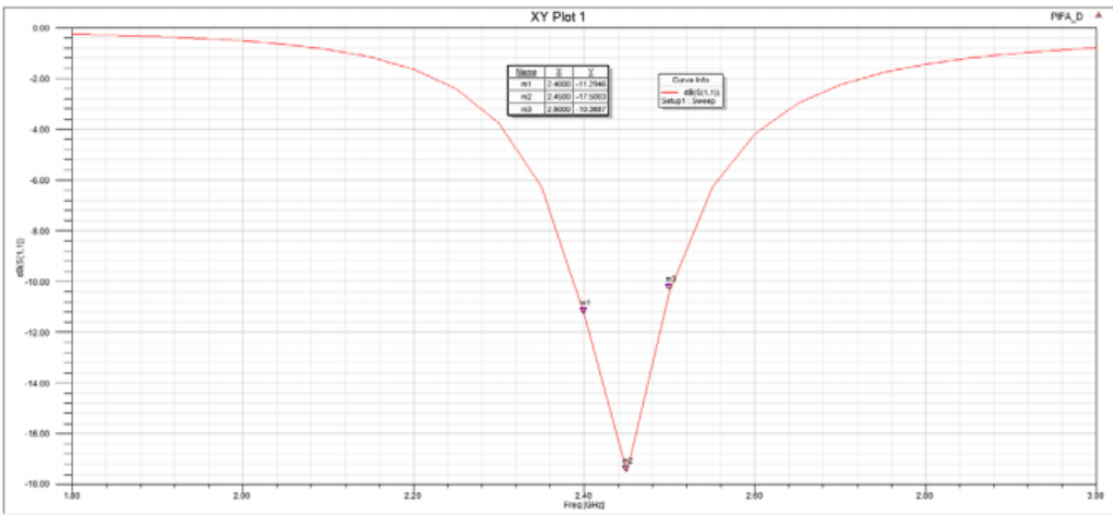
图 1-17 PIFA_D 型天线 S11 参数图
