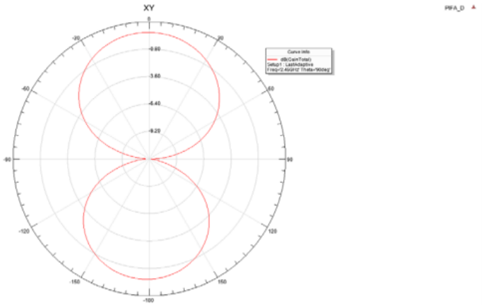
图 1-18 PIFA_D 型天线 XY 面增益图
