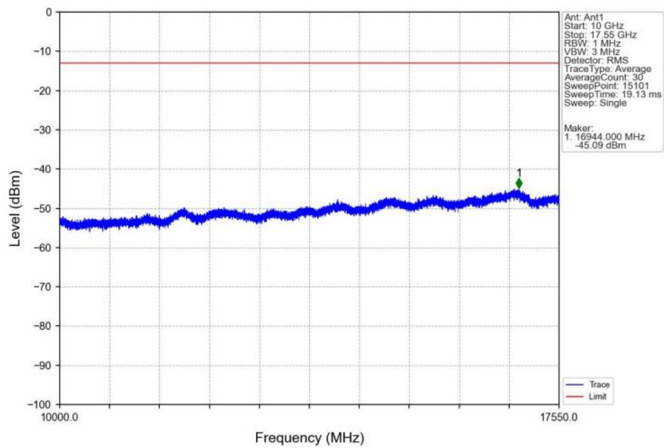
Band4_15MHz_QPSK_LCH_1717.5MHz_RB_1_0_NTNV
