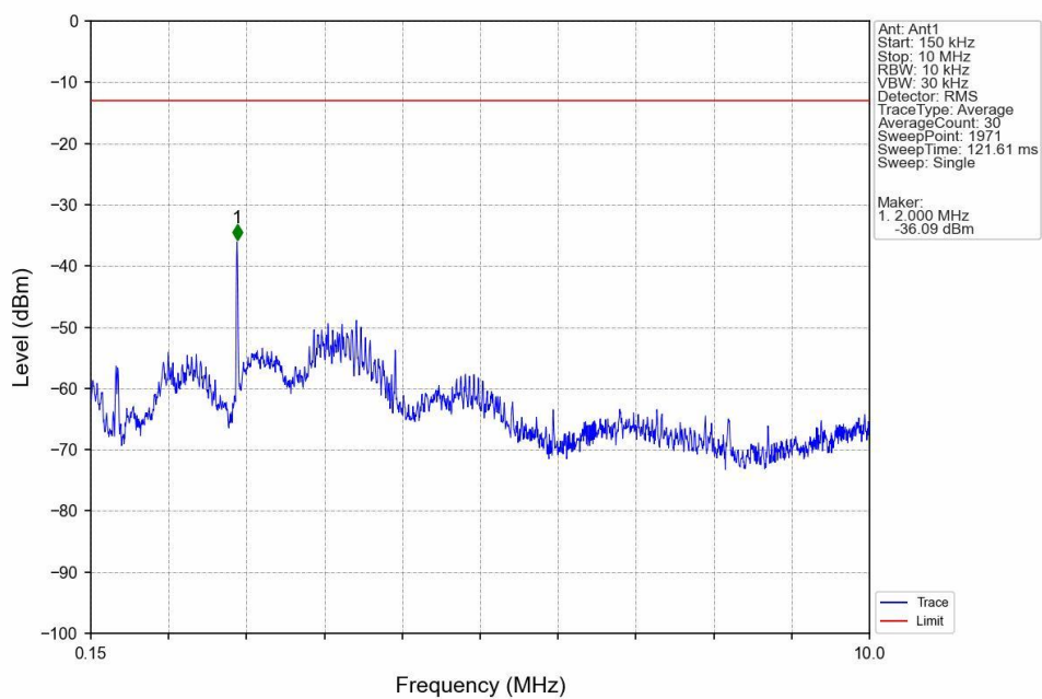
Band2_HSUPA_MCH_1880MHz_Subtest 1_NTNV
