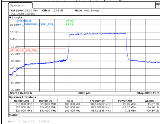
Band 5 10MHz/829.0/Low QPSK 50@0
