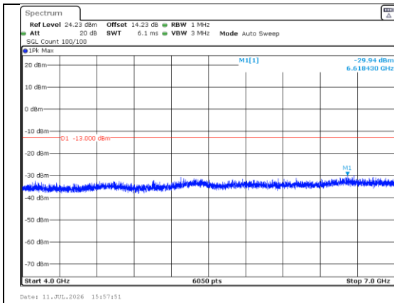
4000.0MHz-7000.0MHz Band 66 5MHz/1712.5/Low QPSK 1@0
