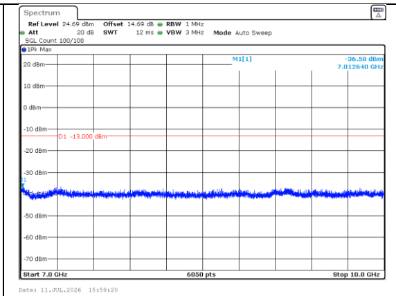
7000.0MHz-10000.0MHz Band 66 5MHz/1712.5/Low QPSK 1@0
