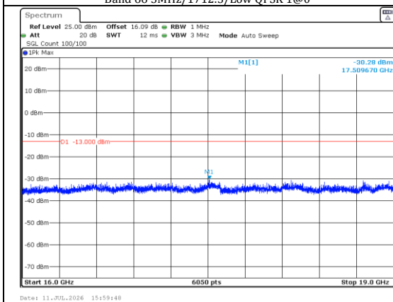
16000.0MHz-19000.0MHz Band 66 5MHz/1712.5/Low QPSK 1@0
