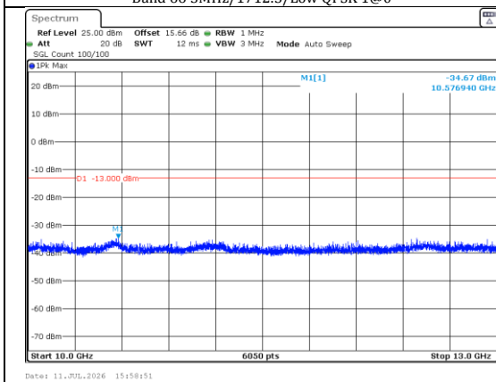
10000.0MHz-13000.0MHz Band 66 5MHz/1712.5/Low QPSK 1@0
