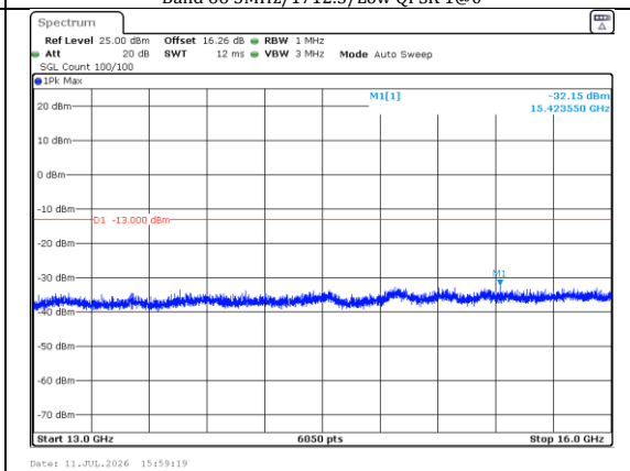
13000.0MHz-16000.0MHz Band 66 5MHz/1712.5/Low QPSK 1@0
