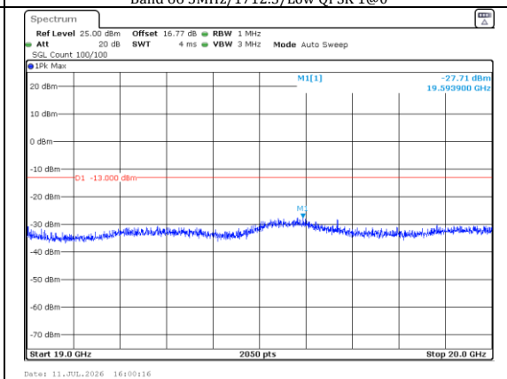
19000.0MHz-20000.0MHz Band 66 5MHz/1712.5/Low QPSK 1@0
