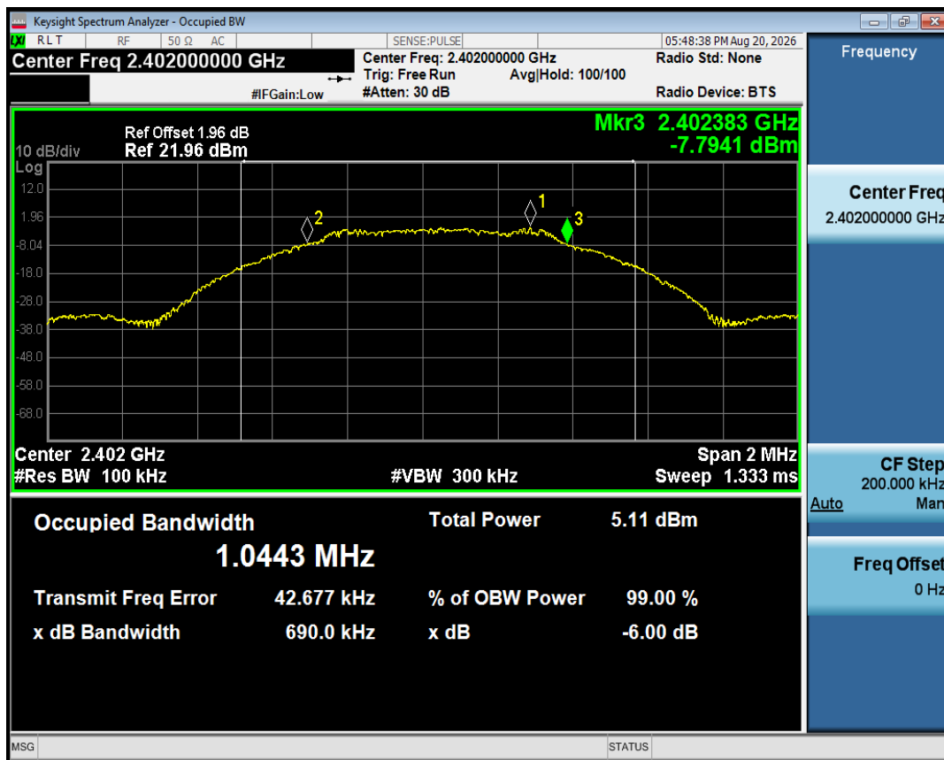
-6dB Bandwidth NVNT BLE 1M 2402MHz Ant1
