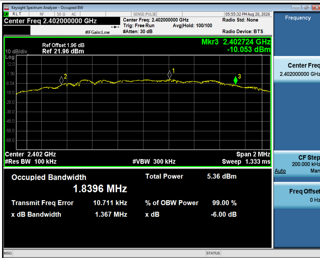
-6dB Bandwidth NVNT BLE 2M 2402MHz Ant1
