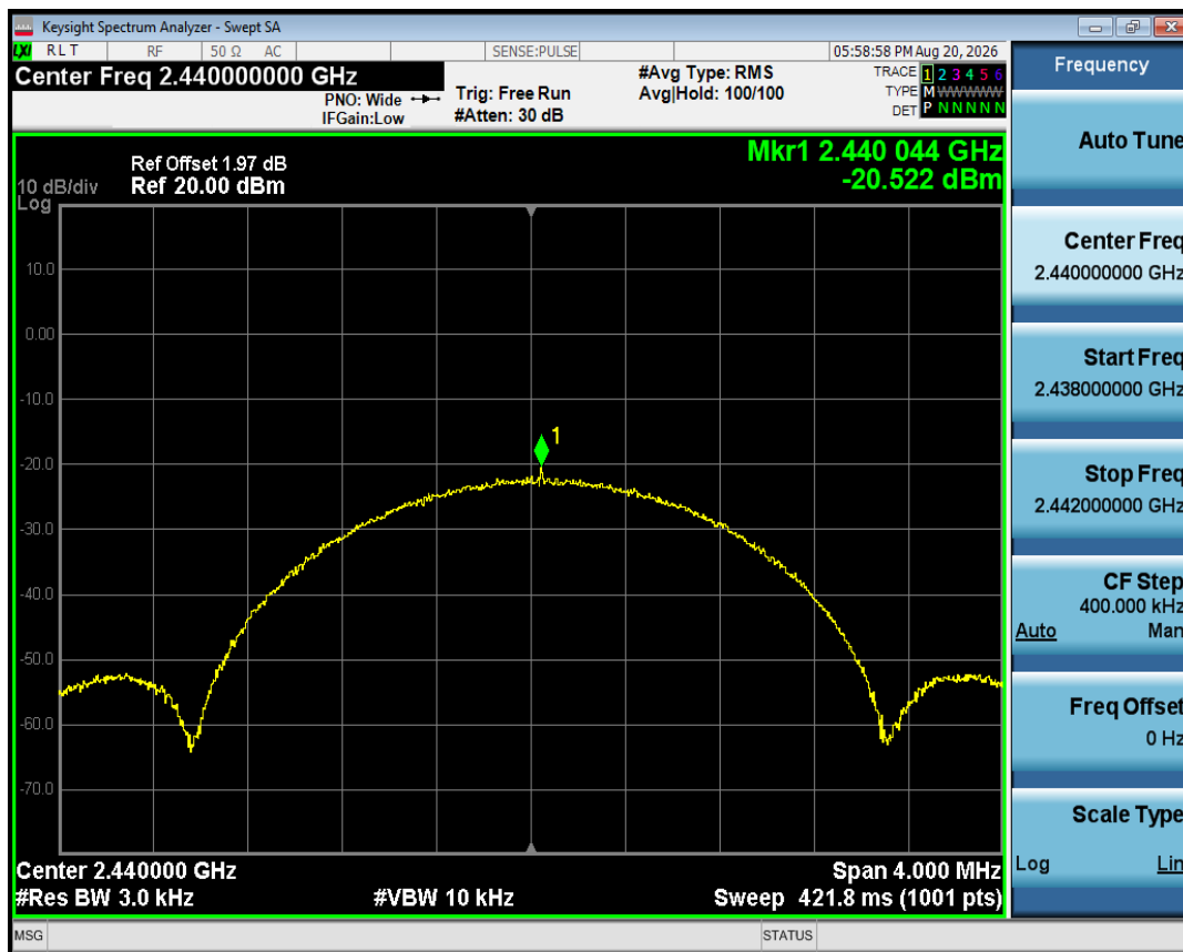
PSD NVNT BLE 2M 2440MHz Ant1
