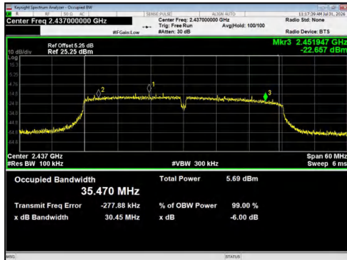
802.11n40 - CH06
