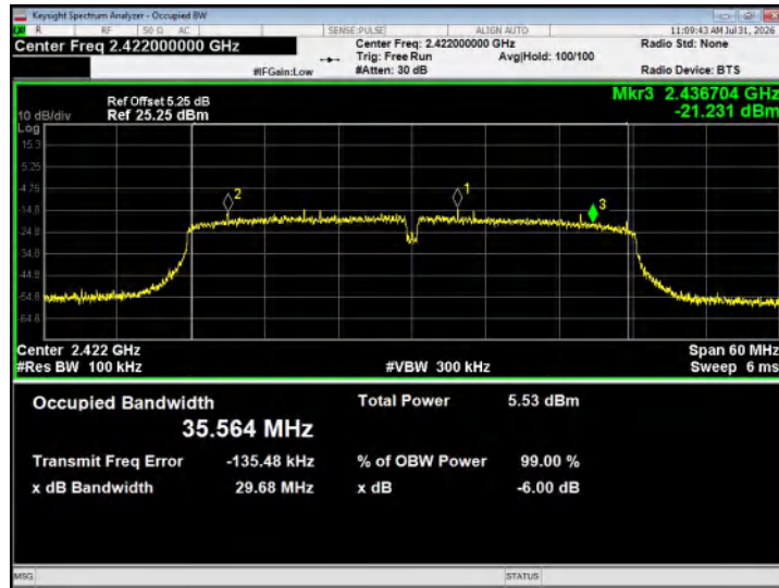
802.11n40 - CH03
