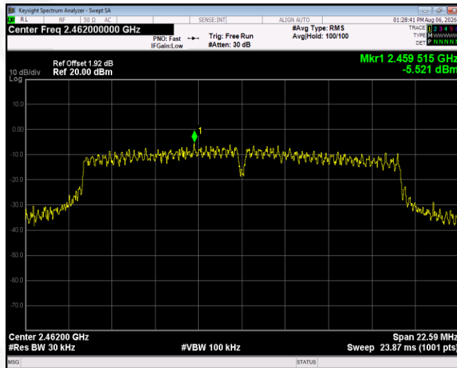
802.11g - CH11
