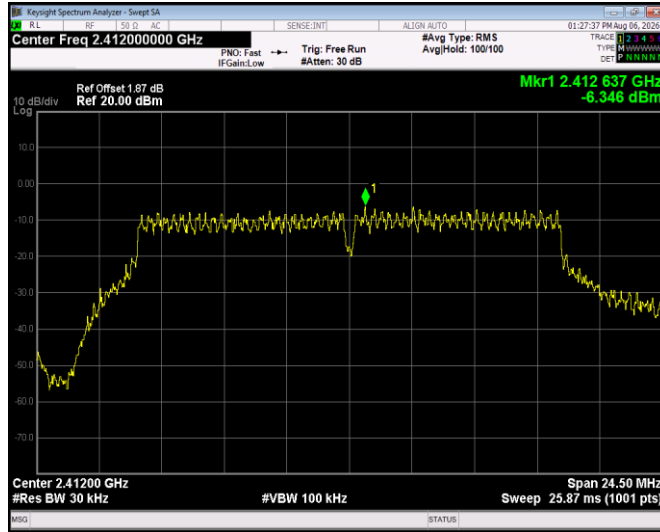
802.11g - CH01
