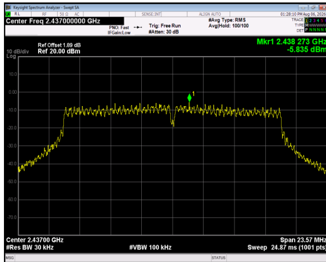
802.11g - CH06
