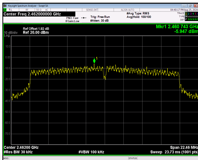
802.11n20 - CH11
