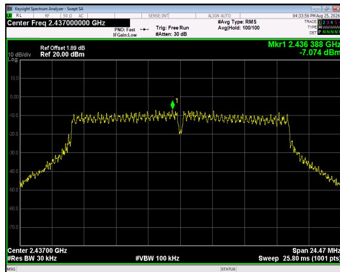
802.11g - CH06
