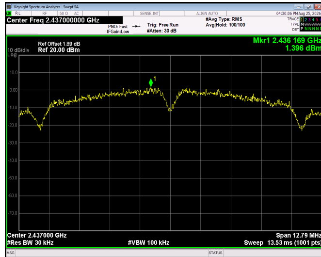
802.11b - CH06
