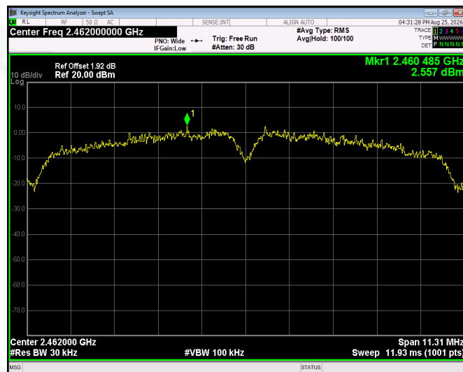
802.11b - CH11
