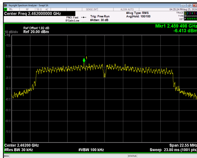
802.11g - CH11
