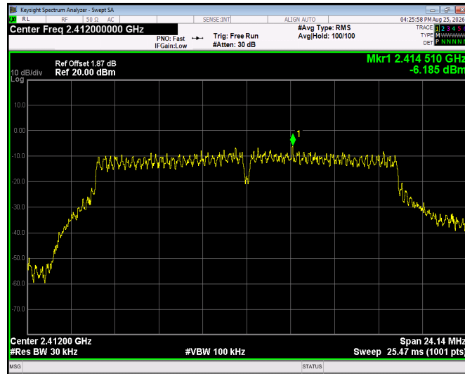
802.11g - CH01
