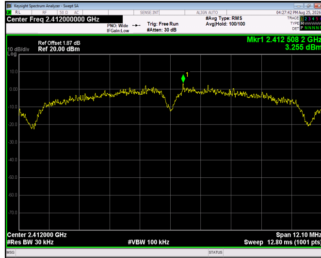
802.11b - CH01
