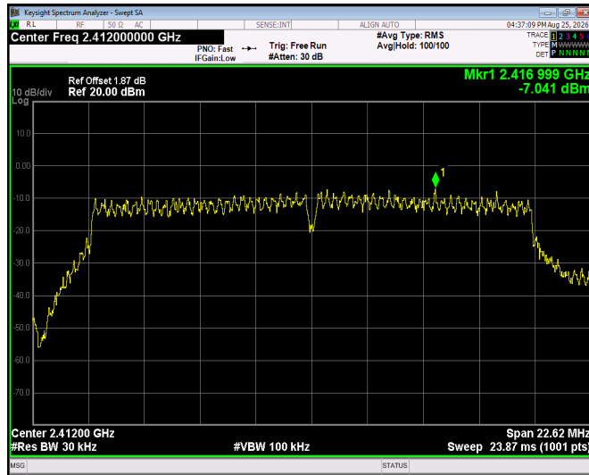
802.11n20 - CH01
