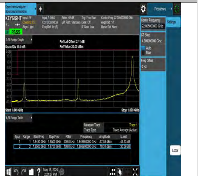
Band2_20MHz_QPSK_18700_1RB#99
