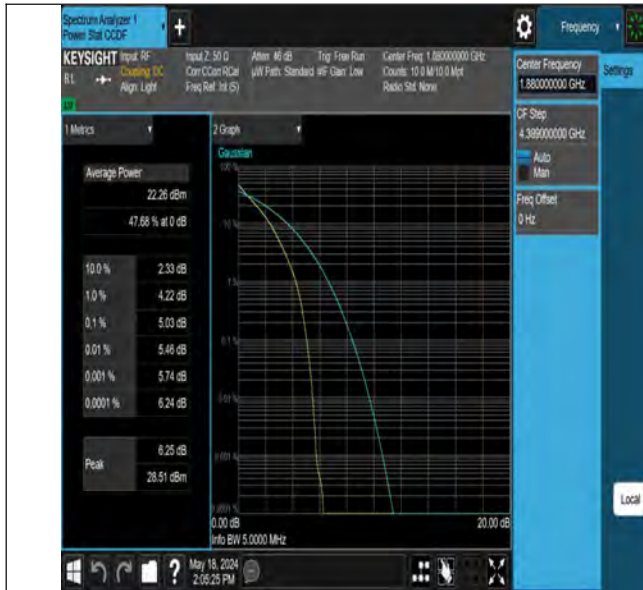
Band2-5MHz-QPSK-18900-25RB#0-PASS
