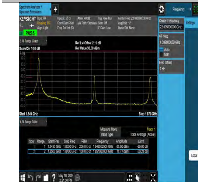
Band2_20MHz_QPSK_18700_1RB#0
