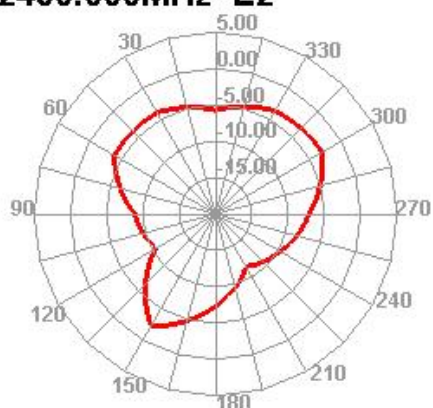
2450.000MHz E2
