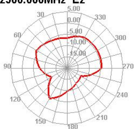
2500.000MHz E2
