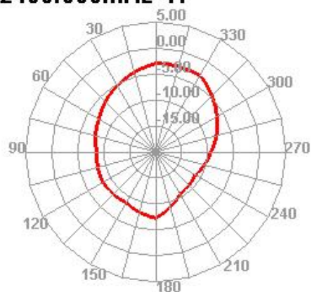
2400.000MHz H
