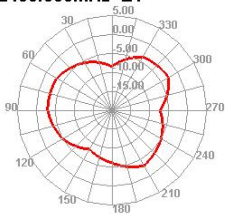
2400.000MHz E1
