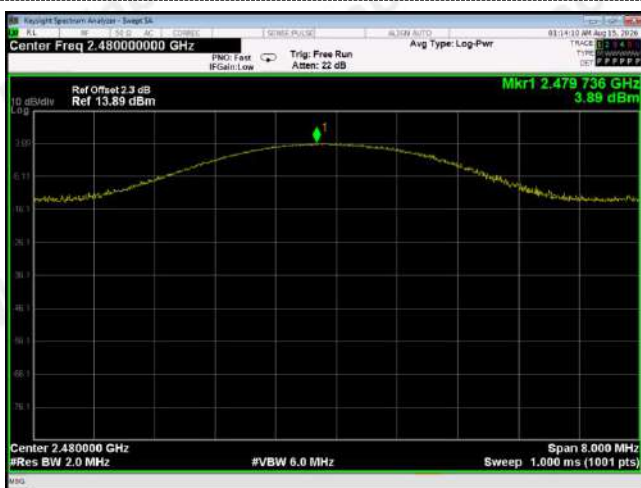
GFSK(CH78)
