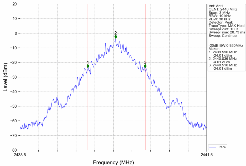
1_MCH_2440MHz_Ant1_NTNV
