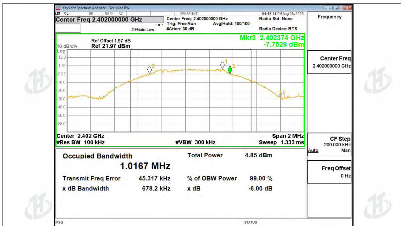
-6dB Bandwidth NVNT BLE 1M 2402MHz Ant1
