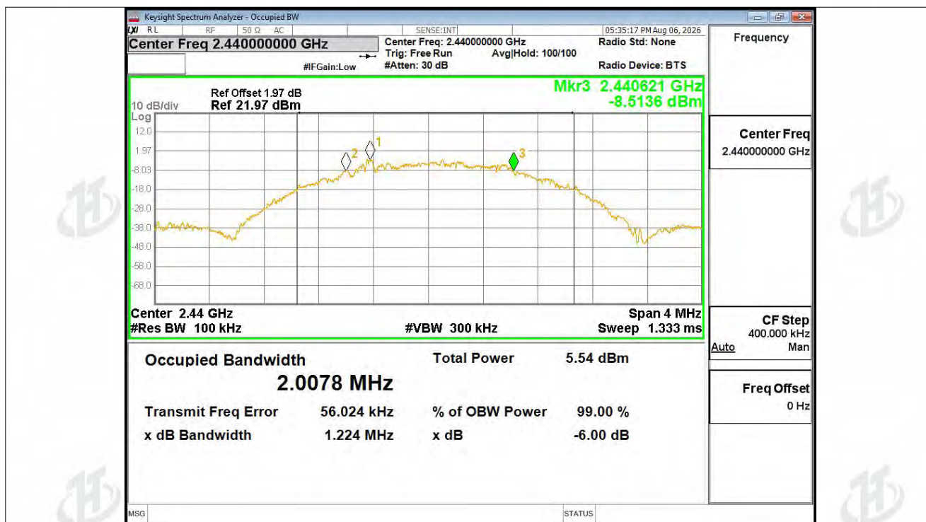
-6dB Bandwidth NVNT BLE 2M 2440MHz Ant1
