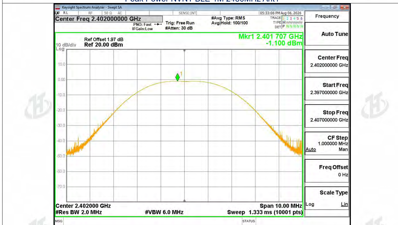
Peak Power NVNT BLE 2M 2402MHz Ant1
