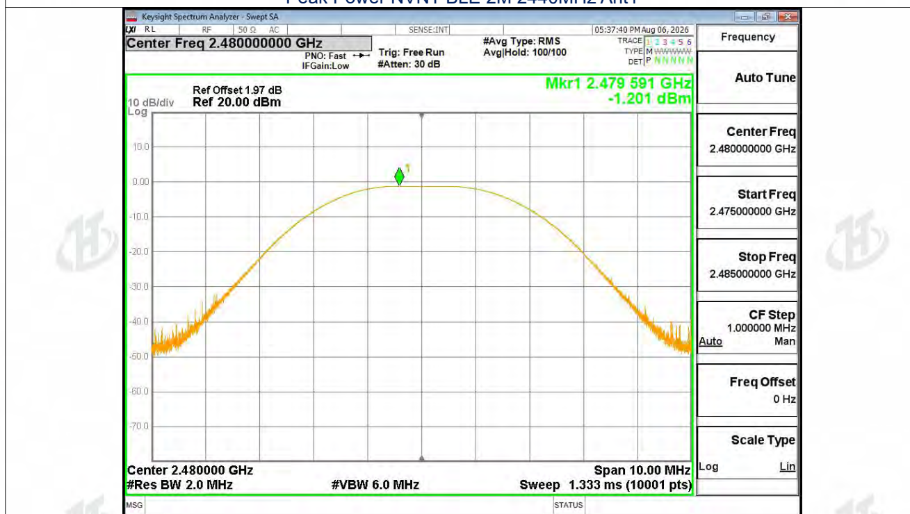
Peak Power NVNT BLE 2M 2480MHz Ant1
