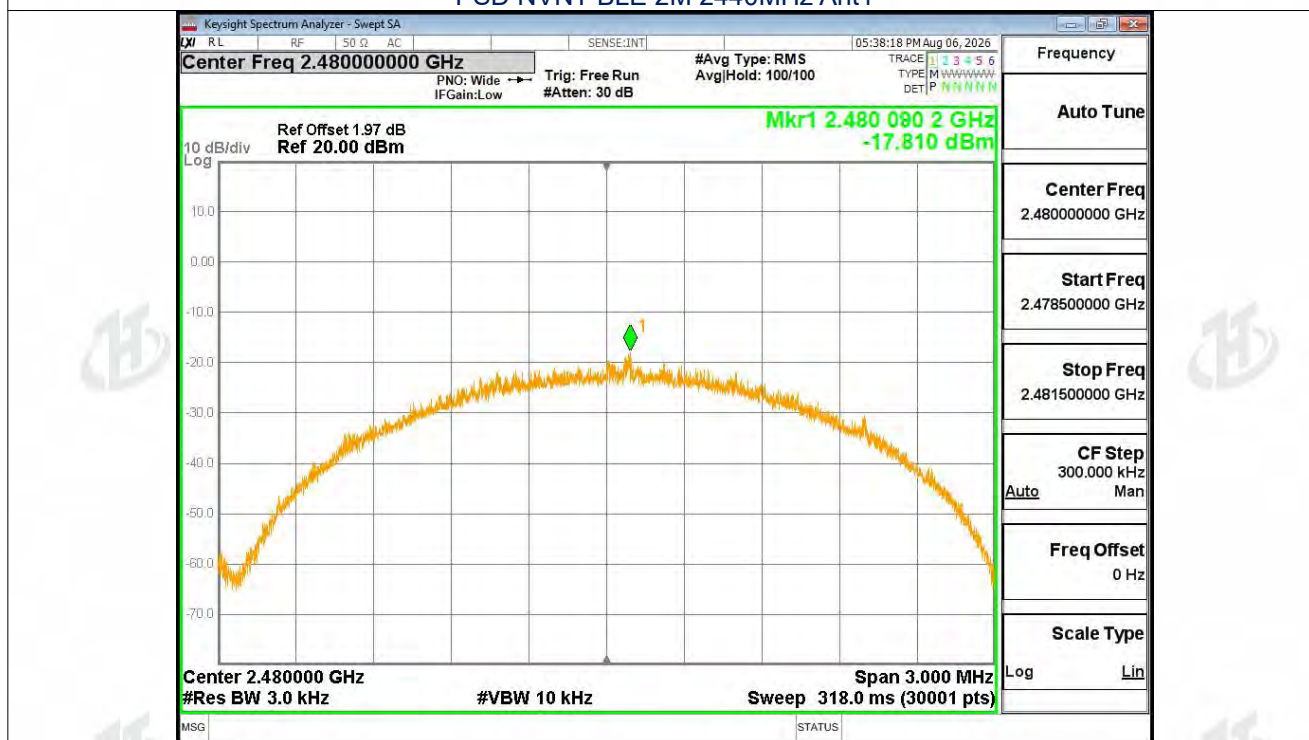
PSD NVNT BLE 2M 2480MHz Ant1
