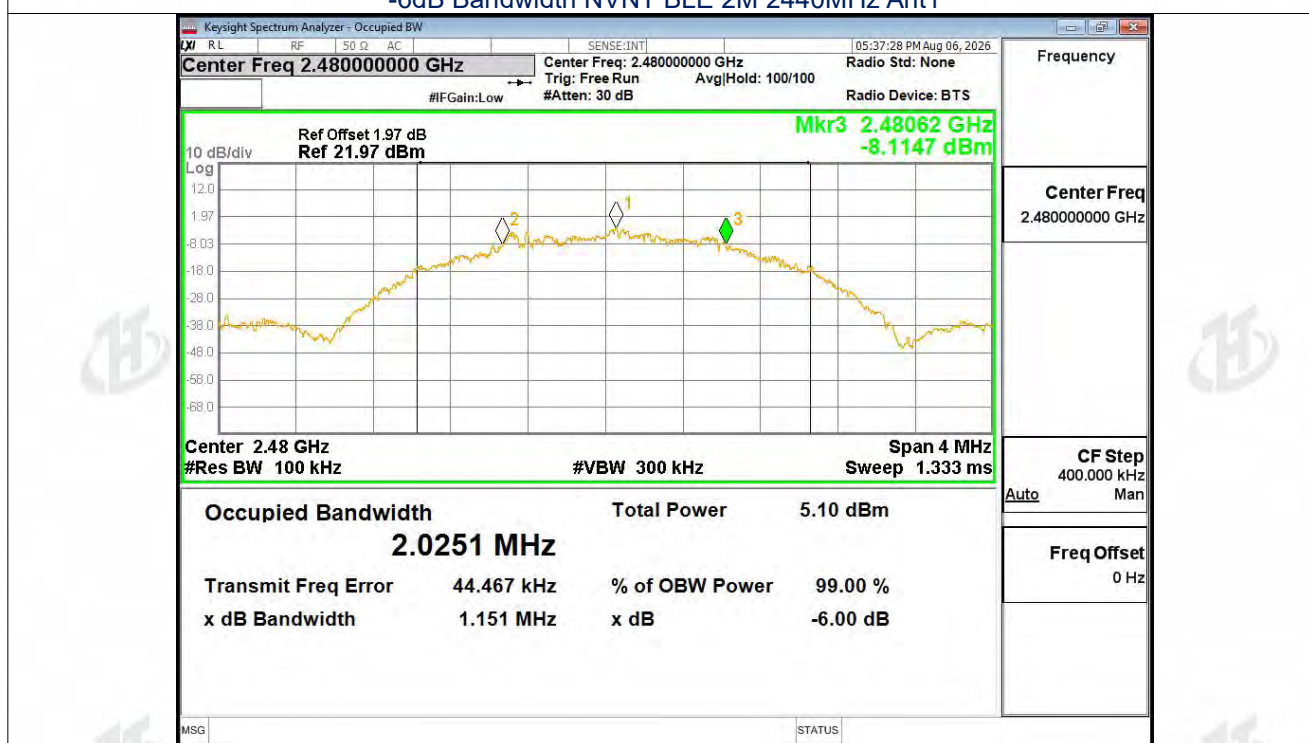
-6dB Bandwidth NVNT BLE 2M 2480MHz Ant1
