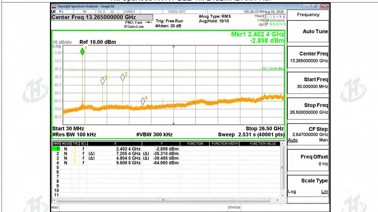
Tx. Spurious NVNT BLE 1M 2402MHz Ant1 Emission
