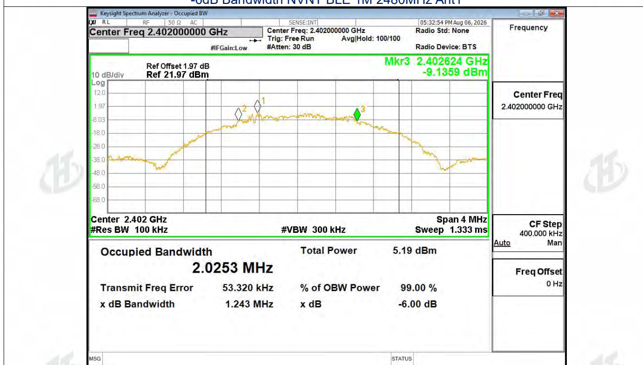
-6dB Bandwidth NVNT BLE 2M 2402MHz Ant1
