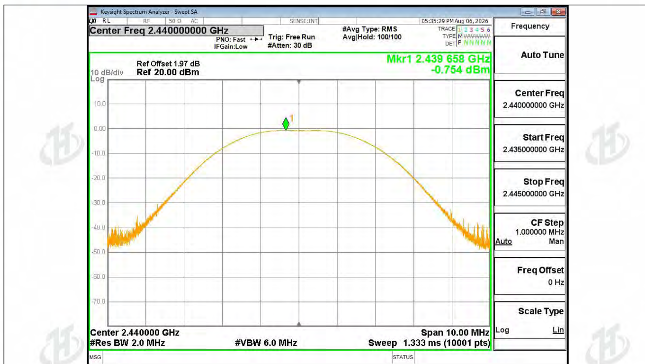
Peak Power NVNT BLE 2M 2440MHz Ant1
