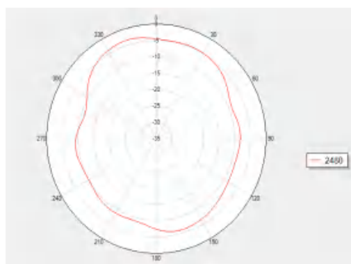
2480MHz XYplane
