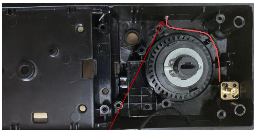
天线贴装位置以及 cable 线走线位置。
