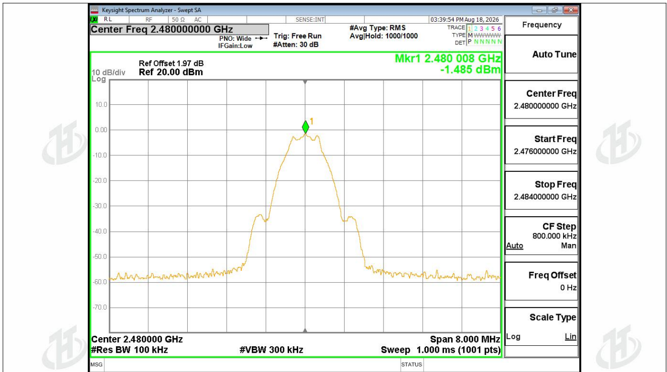
Band Edge NVNT BLE 1M 2480MHz Ant1 Ref
