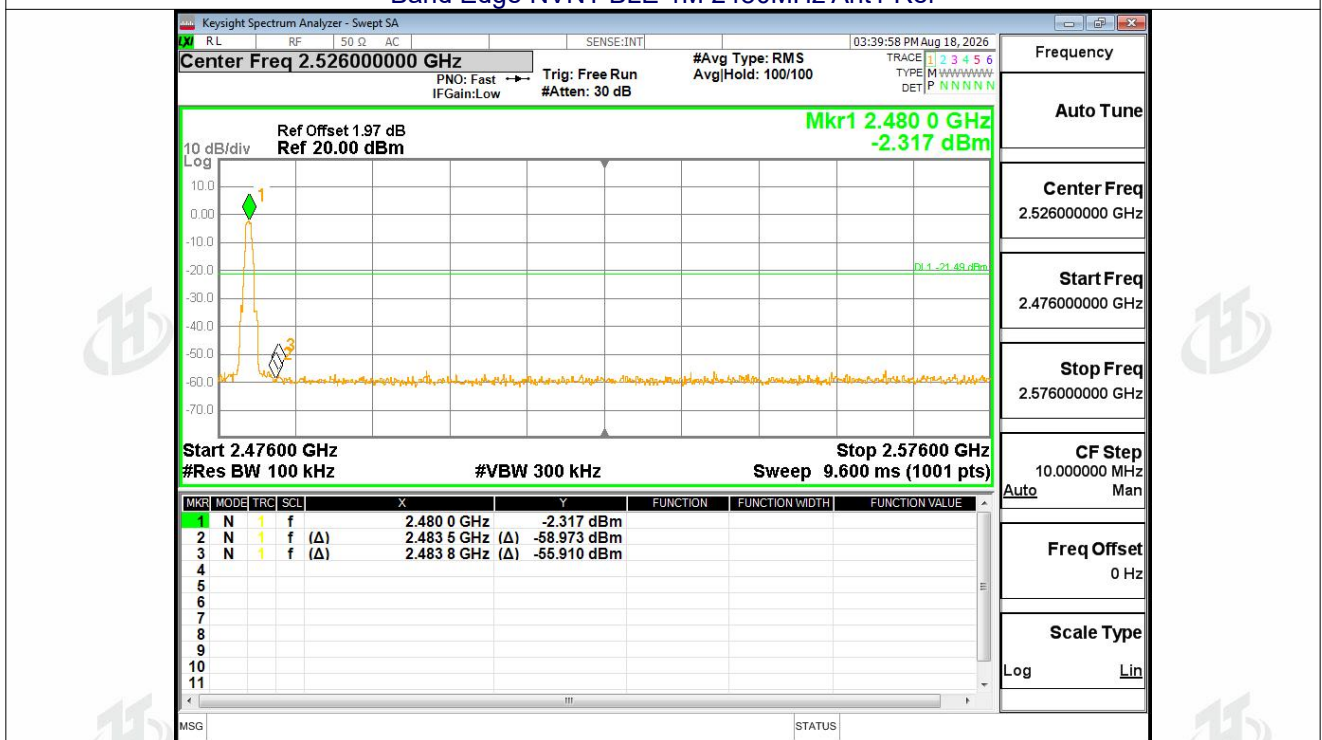
Band Edge NVNT BLE 1M 2480MHz Ant1 Emission
