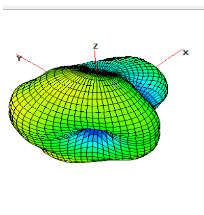
2400MHz
