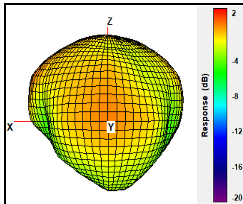
2450MHz
