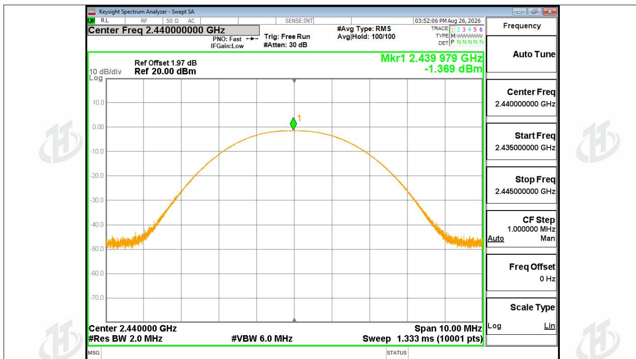
Peak Power NVNT BLE 1M 2440MHz Ant1
