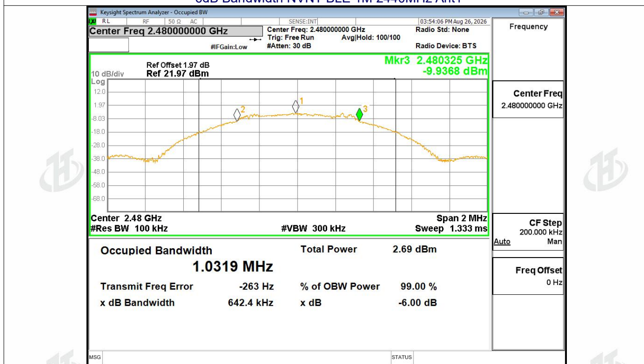
-6dB Bandwidth NVNT BLE 1M 2480MHz Ant1
