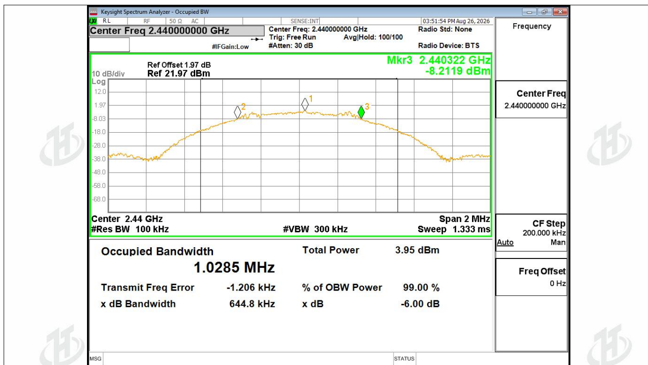
-6dB Bandwidth NVNT BLE 1M 2440MHz Ant1
