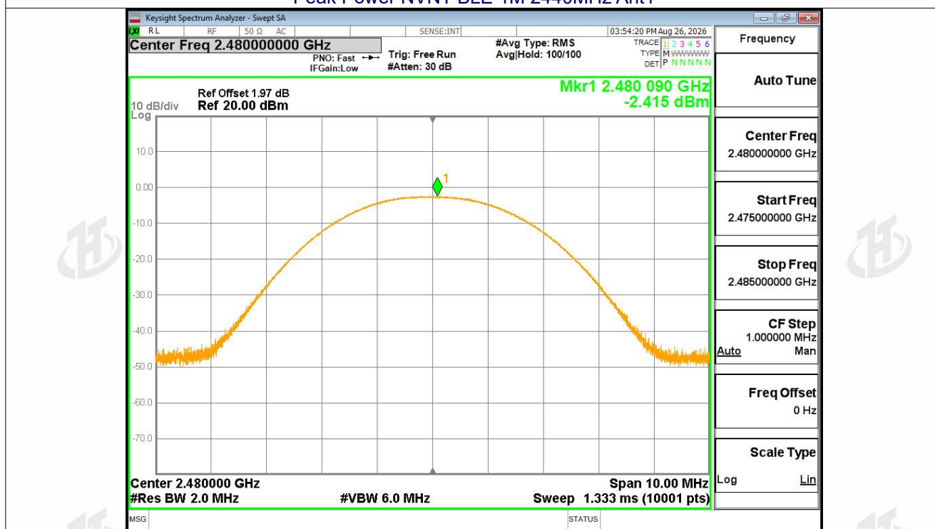
Peak Power NVNT BLE 1M 2480MHz Ant1
