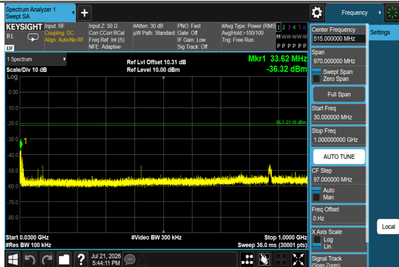
BLE_2M-Ant1-2402-30~1000-PASS
