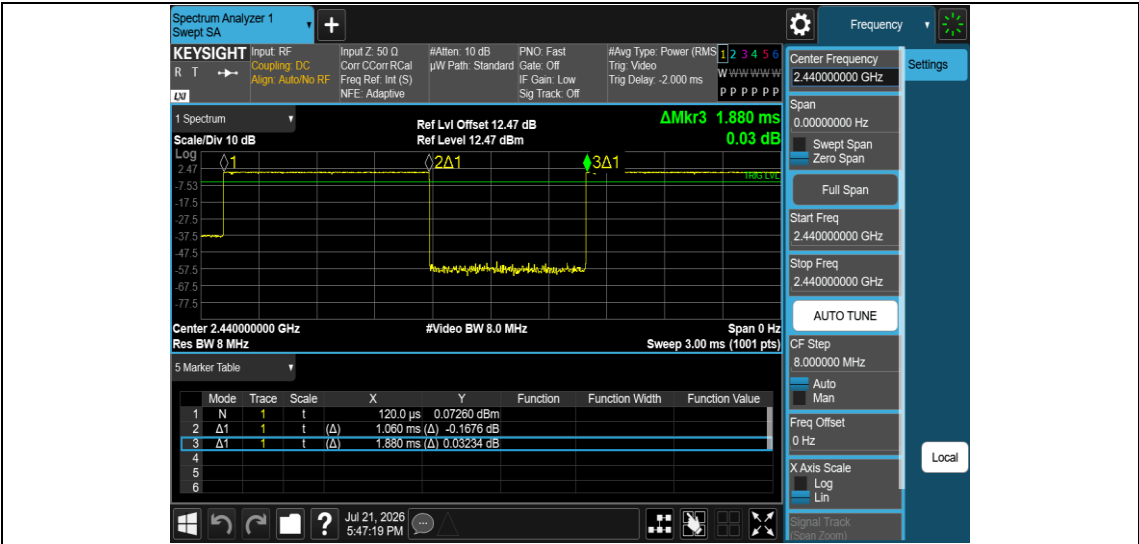
NTNV-BLE_2M-Ant1-2440
