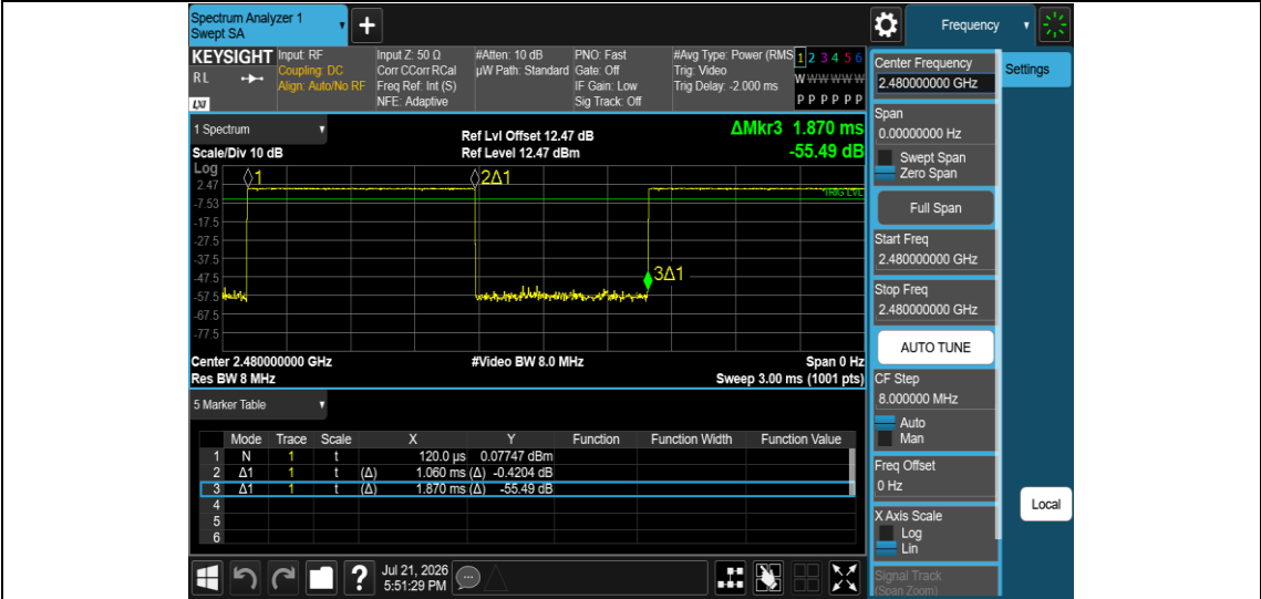
NTNV-BLE_2M-Ant1-2480
