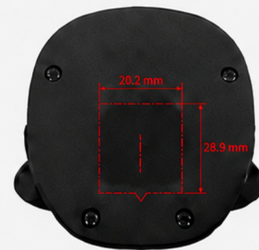
传感器背面（打标位置示意）
