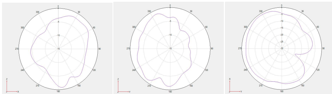
5500MHz (Phi0/Phi90/Theta90)
