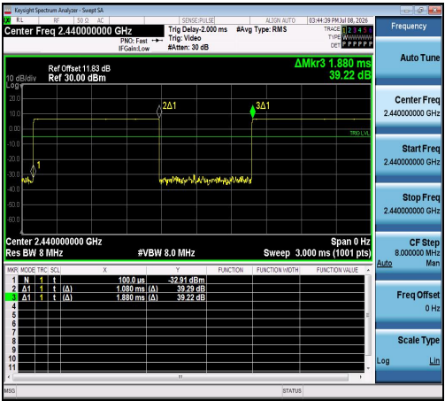
NTNV-LE_2M-Ant1-2440
