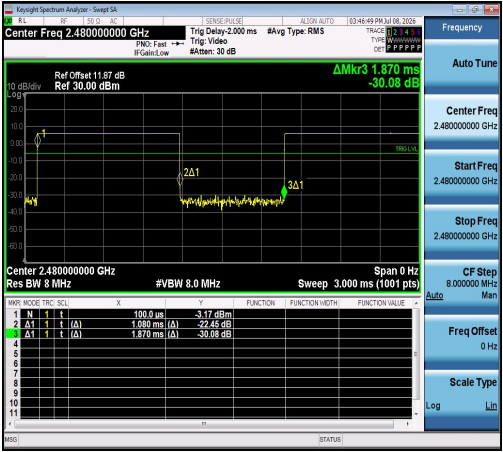
NTNV-LE_2M-Ant1-2480
