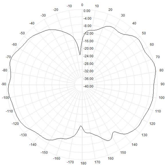
E(928MHz)
