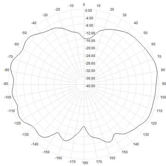
E(915MHz)
