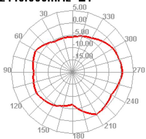
2450.000MHz
