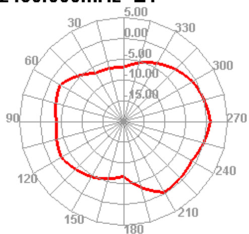
2490.000MHz
