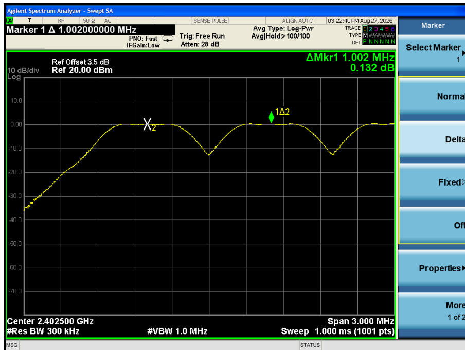
GFSK mode-CH00
